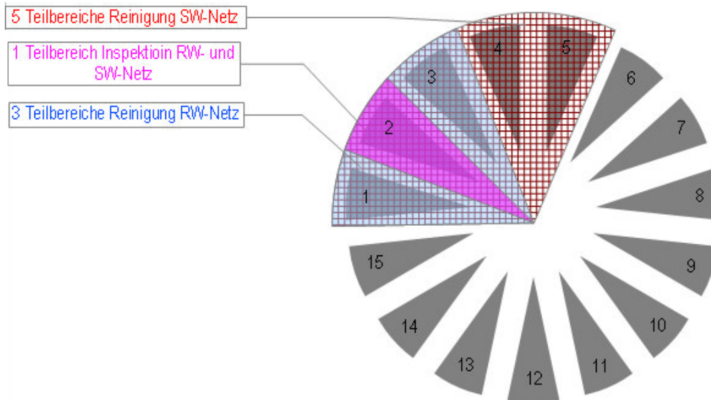
Abbildung 1-1: Jährliche Reinigung und Inspektion bei Netzaufteilung in 15 Teilbereiche
